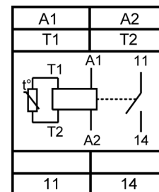
Рис. 2б 24DC
