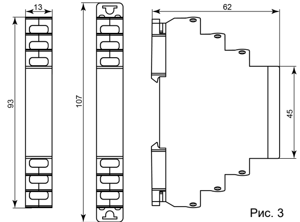
Габаритные размеры
