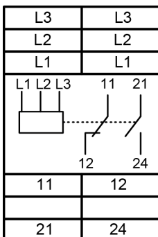
Схема подключения
