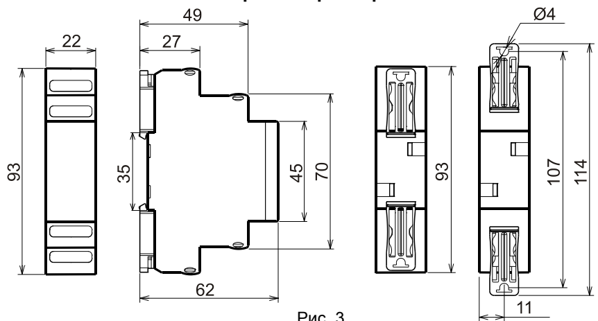
Габаритные размеры
